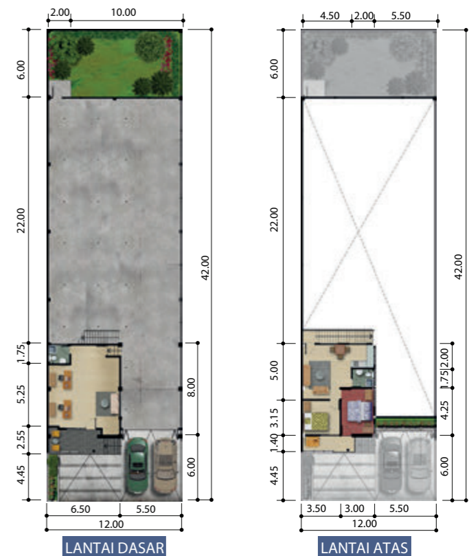
DENAH TIPE STANDAR dengan KANTOR
