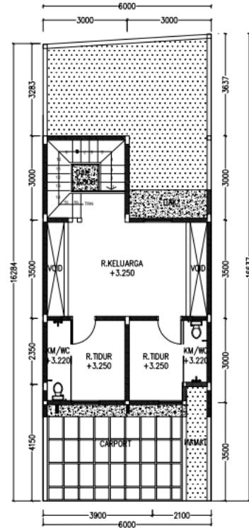
DENAH LANTAI ATAS
